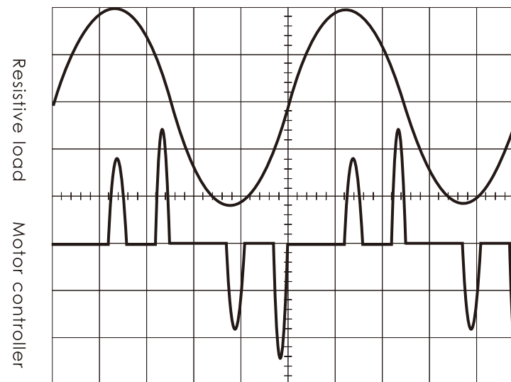
图3：典型的电流波形比较
