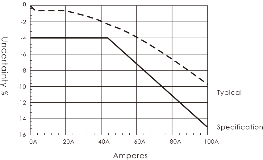
图8: 典型的 DC 信号线性在 10 mV/A 范围时
